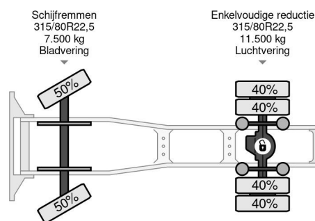
Scania R380 LA 4x2 DAYCAB (EURO 3 / 12 GEARS MANUA...
