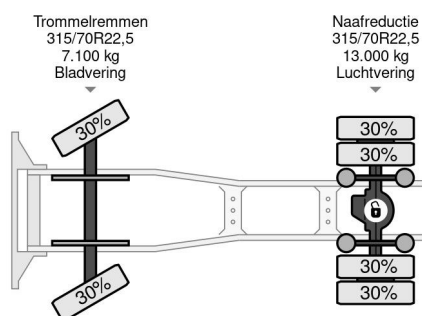
Renault Magnum 430 PRIVILEGE (ZF16 MANUAL GE... 4x2
