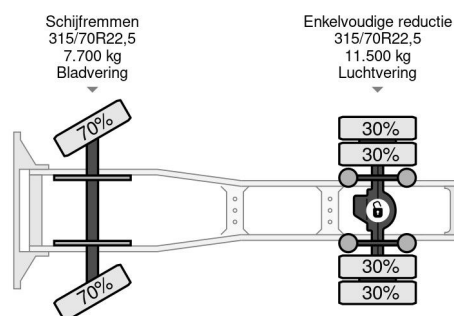
Renault Magnum AE 440 E-TECH (EURO 3 / ZF16 MA... 4x2
